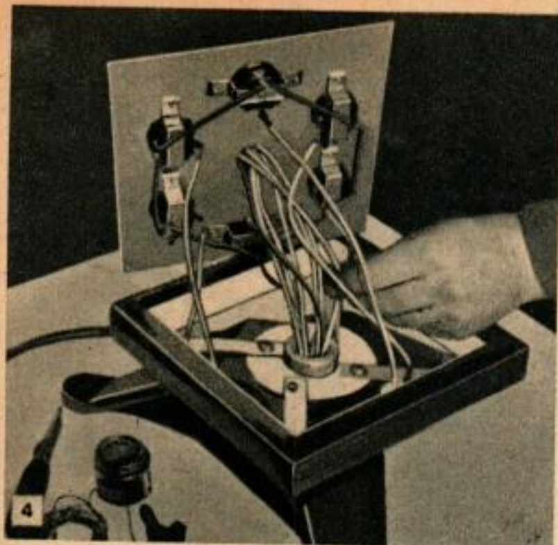
Les prises sont fixées sous le panneau inférieur au moyen de ferrures et les fils passent par le trou central, puis dans la colonne pour atteindre le pupitre.
