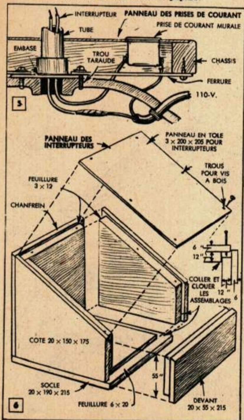
Les prises sont fixées sous le panneau inférieur au moyen de ferrures et les fils passent par le trou central, puis dans la colonne pour atteindre le pupitre.
