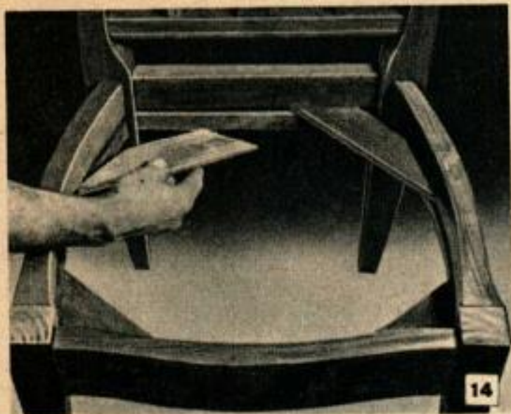
Montage en utilisant un gousset collé entre les rainures pratiquées sur les 4 côtés de la chaise.
