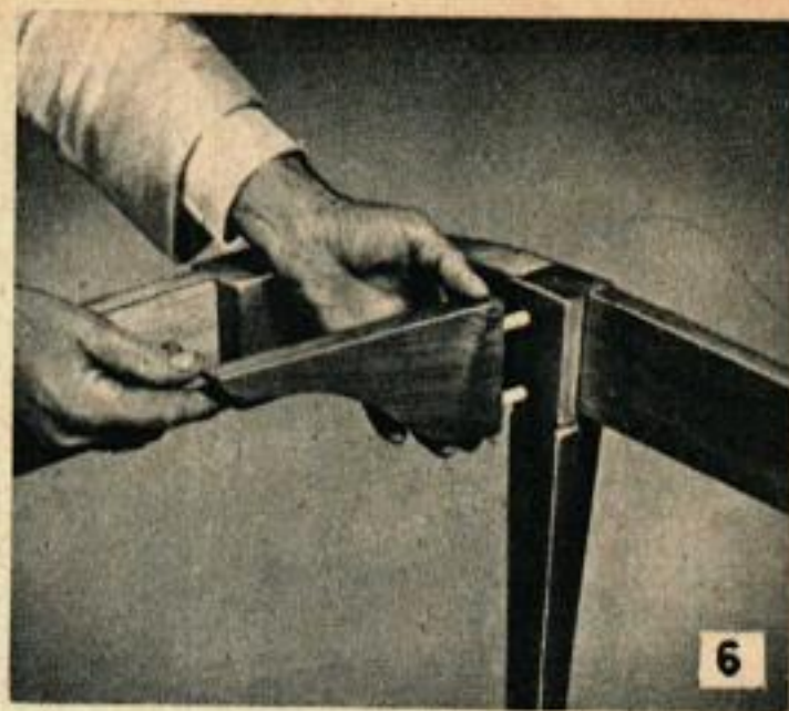
Après collage de la ceinture et des pieds, coller les goussets et serrer à la presse à coller.
