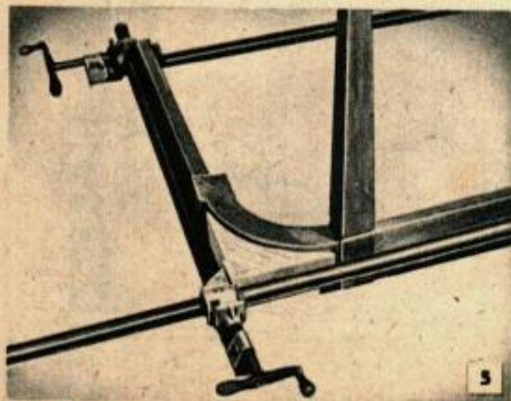
Ci-dessus, essai d'assemblage avant collage afin de vérifier la précision des assemblages, condition d'une bonne rigidité du meuble. Ci-dessous, faire les serrages dans 2 directions à la fois par suite de la présence des coins arrondis.
