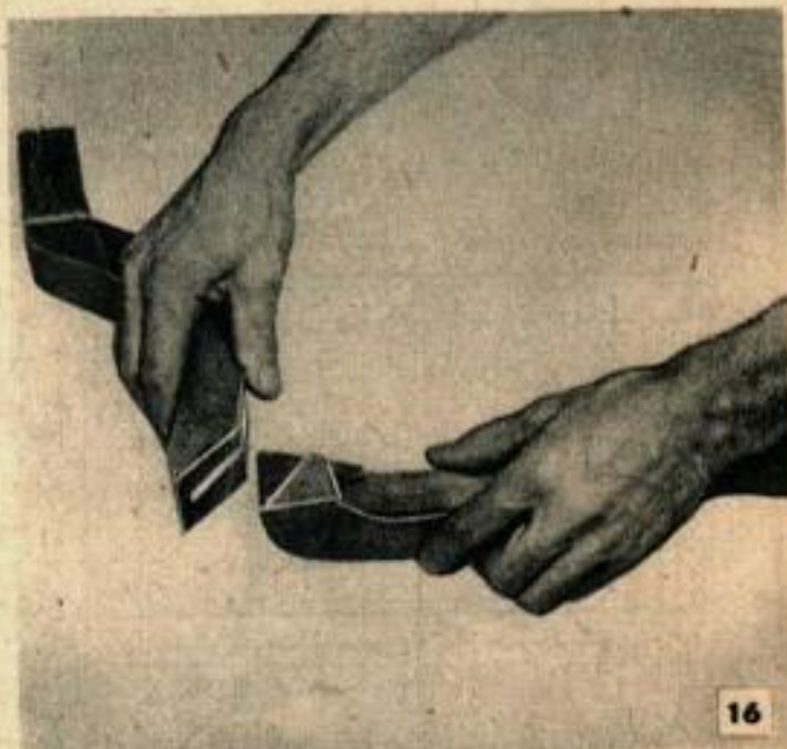
Ci-dessus, les bras en deux pièces du fauteuil ont un assemblage à languette collée donnant plus de rigidité. Ci-dessous assemblage par mortaise et tenon avec le pied arrière et assemblage par vis avec le pied avant.
