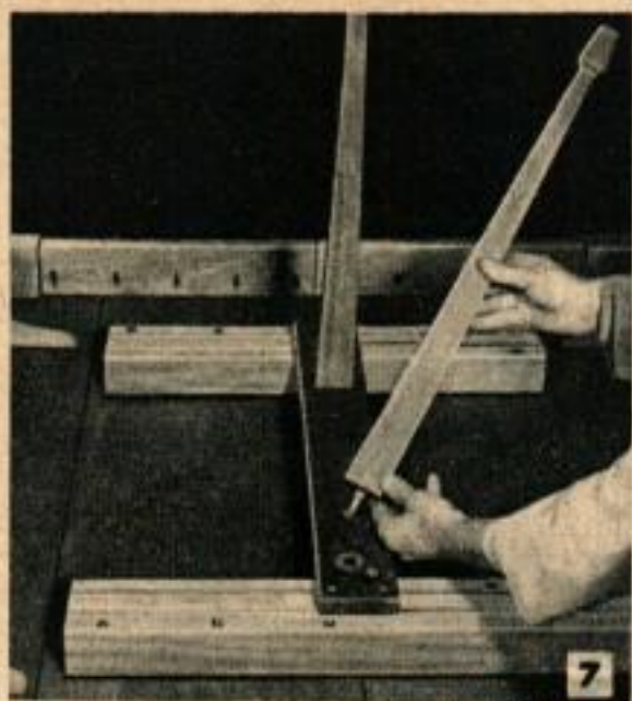
Les pieds du centre sont vissés sur une traverse fixée elle-même sur les coulisses des rallonges. Utiliser des vis à 2 filetages permettant la fixation dans le bout du pied.
