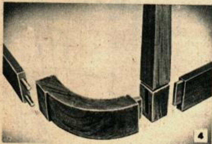
Ci-dessus, essai d'assemblage avant collage afin de vérifier la précision des assemblages, condition d'une bonne rigidité du meuble. Ci-dessous, faire les serrages dans 2 directions à la fois par suite de la présence des coins arrondis.
