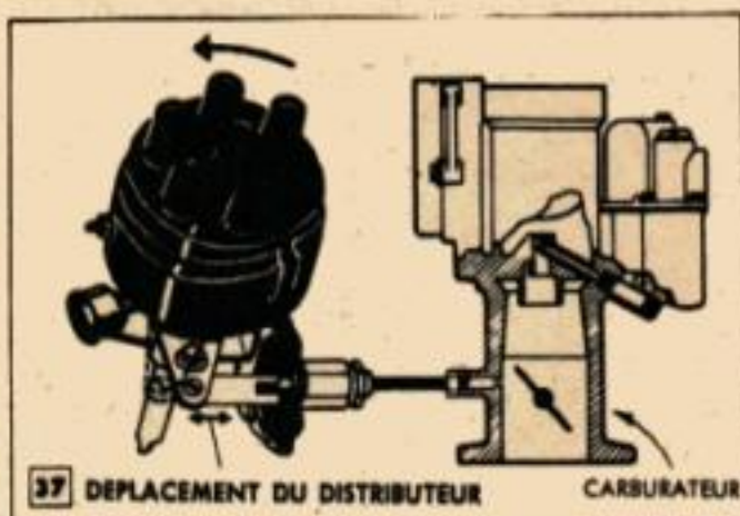
Ci-dessus, réglage de l'avance par l'aspiration du carburateur. Ci-dessous, résultats de l'emploi d'un condensateur trop gros ou trop petit.
