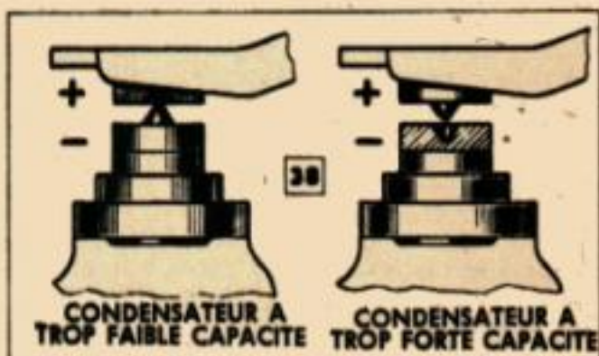
Ci-dessus, réglage de l'avance par l'aspiration du carburateur. Ci-dessous, résultats de l'emploi d'un condensateur trop gros ou trop petit.
