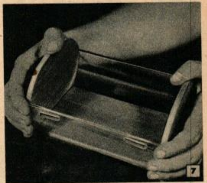
Ci-dessus, les parois sont formées après chauffage autour des deux extrémités et collées sur ces dernières. Ci-dessous les charnières sont pliées, introduites dans les fentes et collées sur le couvercle.
