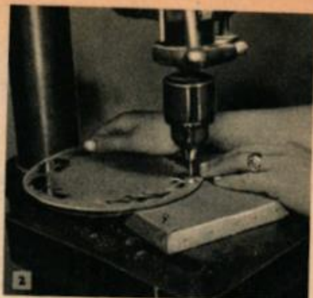
Les motifs décoratifs dépolis améliorent l'aspect du plat à gâteaux. Le dépolissage se fait avec une fraise à bout plat.
