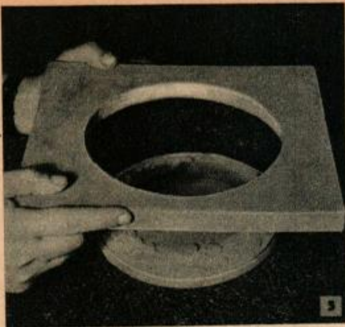
A gauche, emboutissage du couvercle avec des moules en bois.
