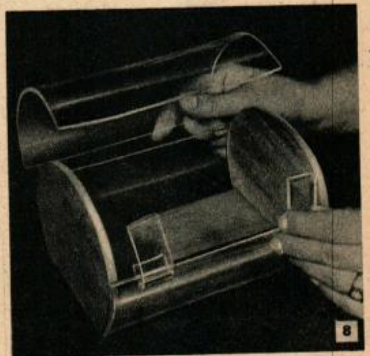
Ci-dessus, les parois sont formées après chauffage autour des deux extrémités et collées sur ces dernières. Ci-dessous les charnières sont pliées, introduites dans les fentes et collées sur le couvercle.
