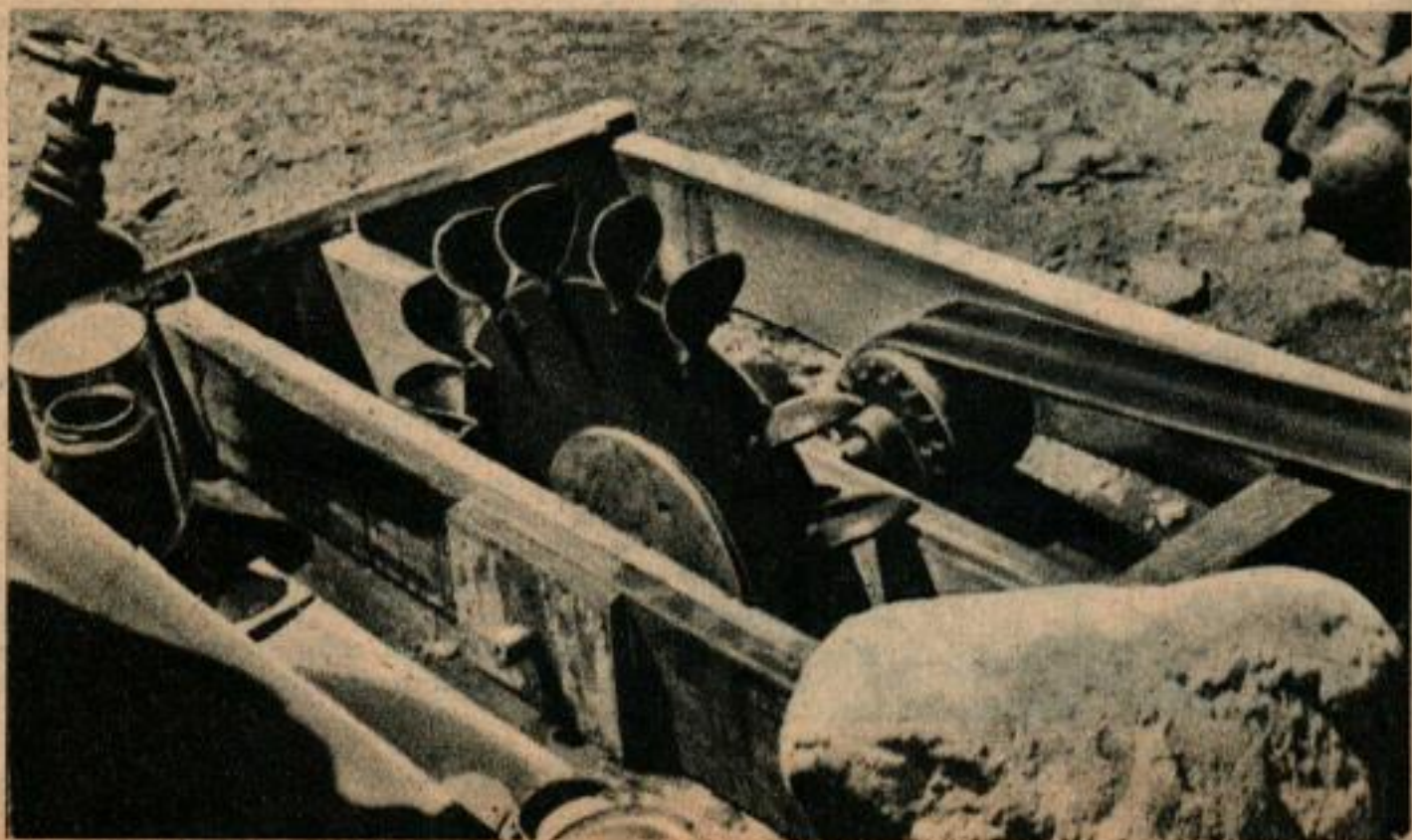
En haut, dessin montrant la disposition de la mine. Ci-dessus, le système à treuil et engrenage a été fait à l'aide d'une vieille boîte de transmission Chevrolet. Ci-dessous, la roue à aube est entraînée par le courant d'eau descendant de la crique où il est prélevé.
