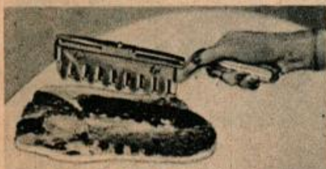
Attendrisseur de beefsteaks. — Il comporte 16 lames qui coupent les tendons sans faire perdre le jus. Une garde limite la profondeur de l'entaille.
