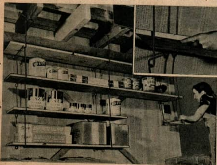
Supports d'étagères ne nécessitant que 4 gros clous pour les tenir. Des planches de plus de 30 cm de large sont placées en travers de ces supports. Les étagères inférieures sont suspendues aux supports déjà en place.
