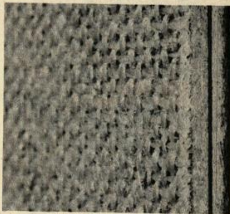
RAINURE SUR CHANT AGRANDIE 2 FOIS REVÊTEMENT TOILE DE JUTE ISOREL.
