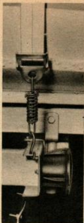
LE SPARE-N-DOLLY sert à deux choses : fixer la roue de secours, et s'en servir pour faciliter les manœuvres des remorques et des bateaux. Il est fabriqué en plusieurs tailles.
