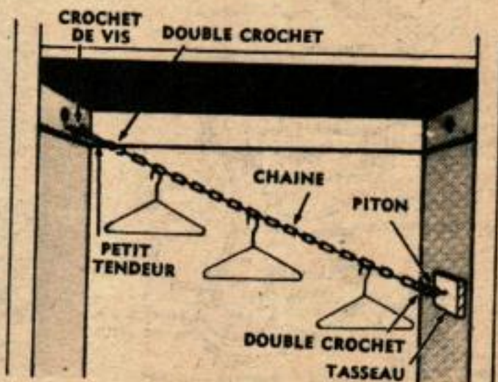
UNE CHAÎNE DE PENDERIE à la place de la tringle est très pratique s'il y a des enfants d'âges différents dans la maison. On place le tasseau de façon à mettre un bout à la portée du plus petit et on tend la chaîne avec le tendeur.
