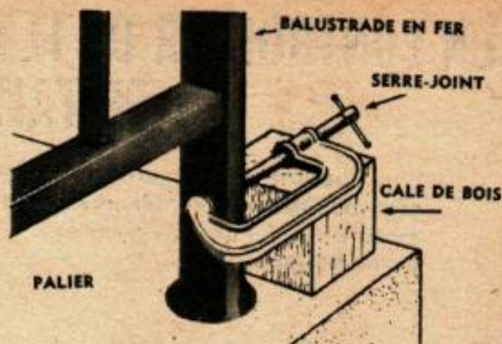
QUAND ON INSTALLE UNE BALUSTRADE décorative en fer sur un perron en béton, verrouiller un serre-joint sur le pilier et utiliser une cale de bois pour caler ce dernier à la hauteur désirée dans le trou avant de couler du plomb fondu autour de la base.
