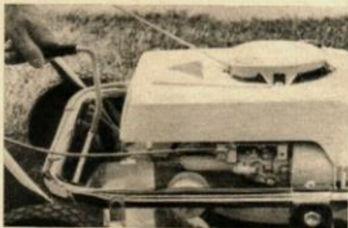
La construction « monorail » de la tondeuse Homko permet de lever et de baisser d'un même levier le châssis et la lame. Le guidon comporte une trousse à outils.
