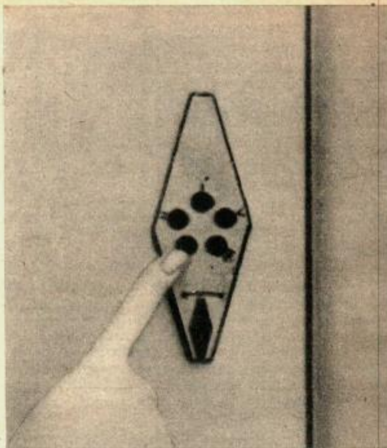
La serrure « Simplex » s'ouvre en poussant par exemple trois boutons dans un certain ordre. On tourne ensuite la petite poignée à droite pour dégager le verrou.
