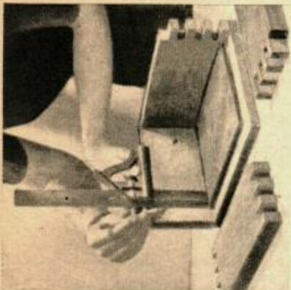
Pour avoir un joint parfait au dernier coin, faire correspondre la profondeur des créniaux coupés à la main à la feuillure du couvercle.
