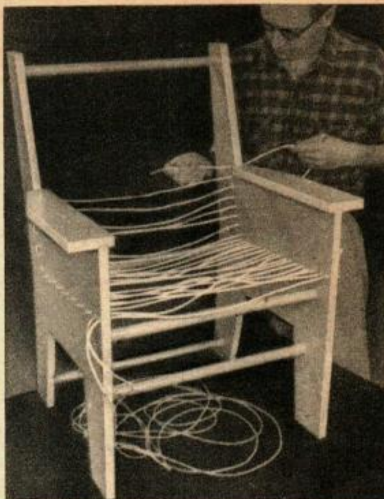
LES CINQ MONTANTS en rondin de 50 cm sont fixés aux flasques par des trous avec de la colle et des vis.
