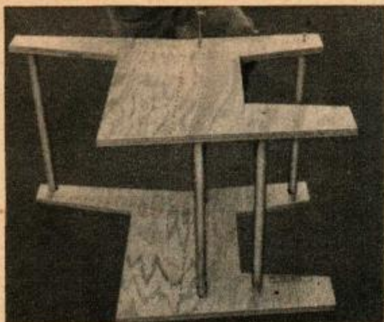
LES CINQ MONTANTS en rondin de 50 cm sont fixés aux flasques par des trous avec de la colle et des vis.
