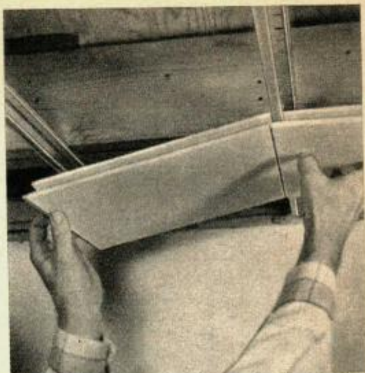
Le joint à languette et rainure entre les carreaux dissimule l'aile de la baguette métallique en Z sur laquelle le plafonnage est posé.
