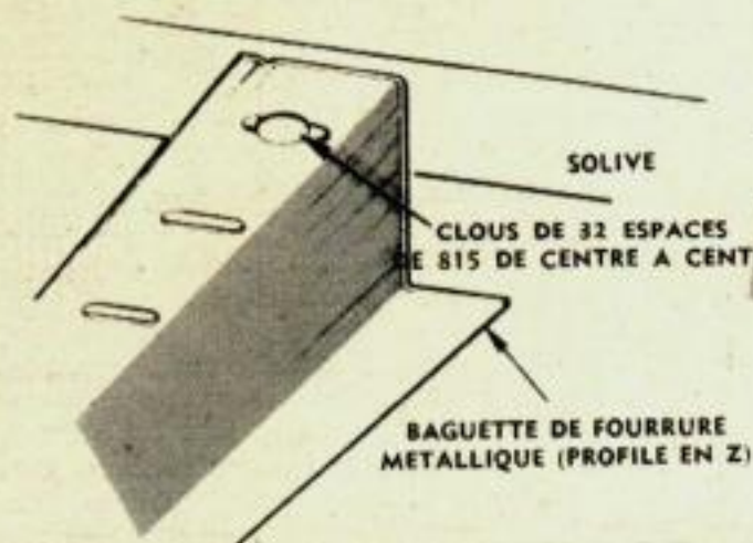
L'installation des baguettes de fourrure métalliques ultra-légères est plus facile que le clouage de planches de fourrure ordinaires.
