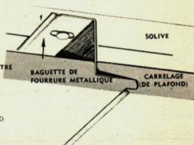
Le joint à languette et rainure entre les carreaux dissimule l'aile de la baguette métallique en Z sur laquelle le plafonnage est posé.
