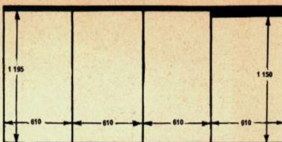
PLAQUE DE FIBRE DURCIE DE 3 × 1 220 × 2 440 2 PIÈCES
