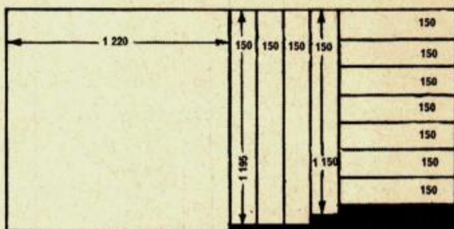
DIAGRAMME DE COUPE DES PANNEAUX
