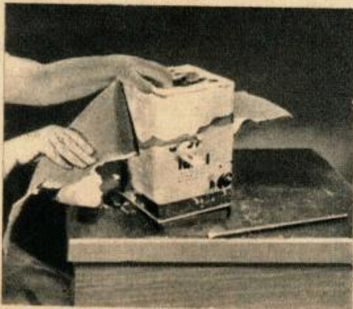
Ci-dessus, le modelage du plâtre à la main dans un moule fait d'une boîte en carton. Ci-dessous, lorsque le plâtre a pris, déchirer la boîte. À droite, lisser le dessus de la pièce coulée avec une lime et du papier de verre.
