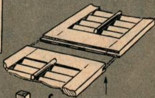
METHODE DE JOINTAGE VERTICAL DE DEUX VOILETS
