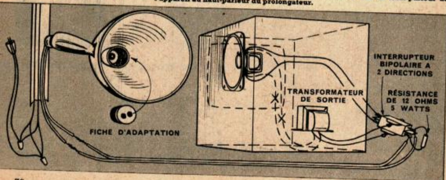
Une fiche d'adaptation, un haut-parleur et un habillage décoratif à grille remplacent l'ampoule d'éclairage. Le frottement maintient le tout en place.
