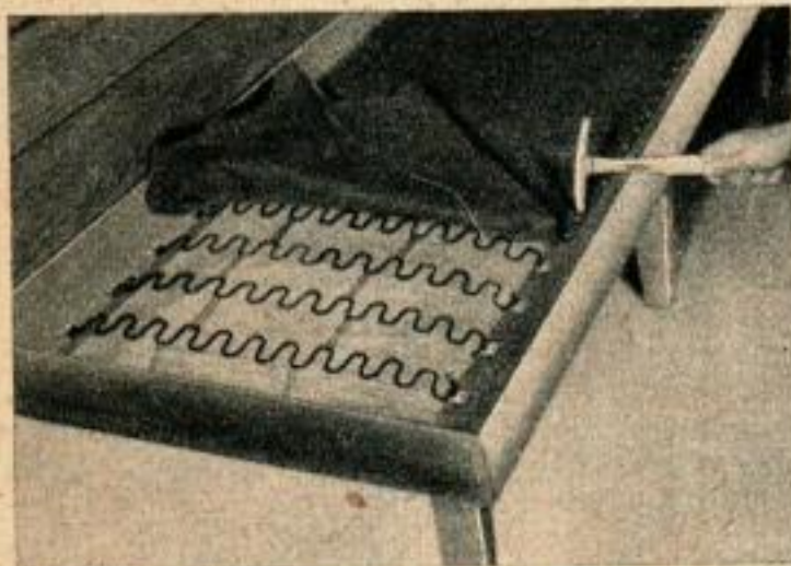
Ci-dessus : lorsque le cadre a été garni de ressorts du type illustré ici, ceux-ci sont recouverts de treillis. Ci-dessous : des chutes de caoutchouc-mousse collées les unes aux autres peuvent être utilisées pour confectionner le rembourrage des coussins.
