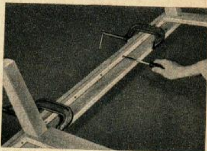
Ci-dessus : des vis enfoncées à travers les tasseaux de dessous servent à assembler les éléments avant et arrière. Ci-dessous : les vis fixant les planches du dossier sur les montants sont chambrées, leur tête est chevillée et les chevilles sont poncées à fleur du bois.
