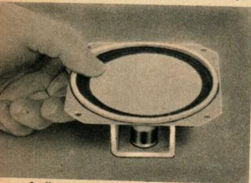
Le disque en carton bristol est collé à la colle caoutchoutée sur le cône du haut-parleur, juste à l'intérieur de la partie ondulée de celui-ci.
