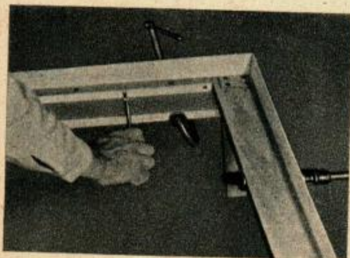
Ci-dessus : de la colle et plusieurs longues vis sont employées pour ancrer solidement les pieds de devant. Ci-dessous : des vis enfoncées à travers les tasseaux de dessus servent à la fixation des planchettes de bordure de l'encadrement.
