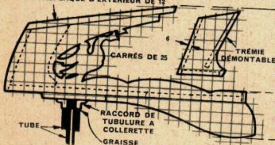
MANGEOIRE PIVOTANTE
