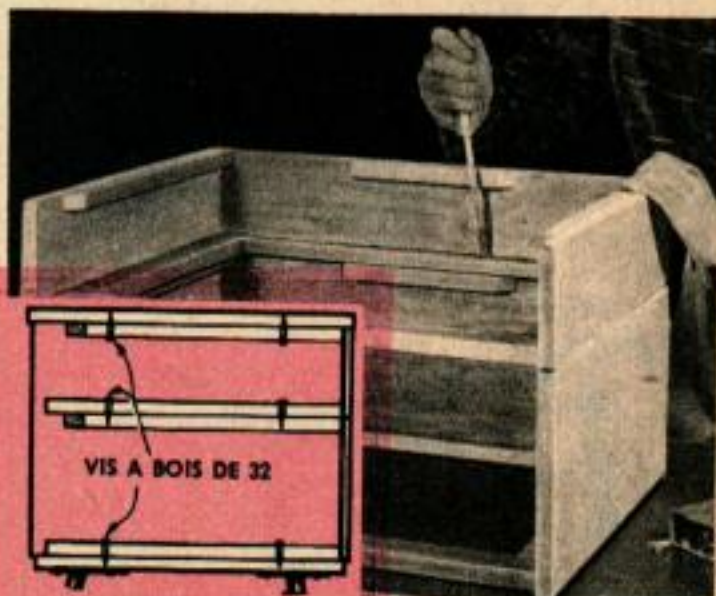
Qu'ils soient disposés l'un au-dessus de l'autre ou l'un à côté de l'autre, les éléments à tiroirs sont assemblés par des vis traversant les cadres.
