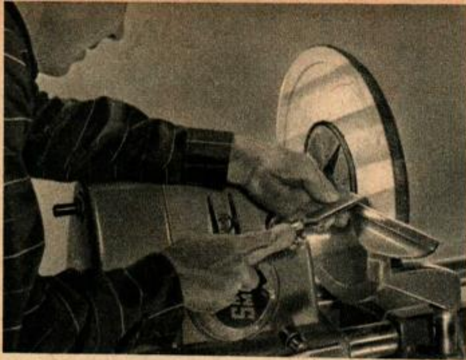
Photo du haut à droite: le tabouret de coiffeuse modèle «étal de boucherie» est confectionné par collage de planches de bois dur de grain et couleur contrastants. La photo de gauche montre comment le fond du siège est tourné en oblique afin de donner une inclinaison suffisante aux pieds.
