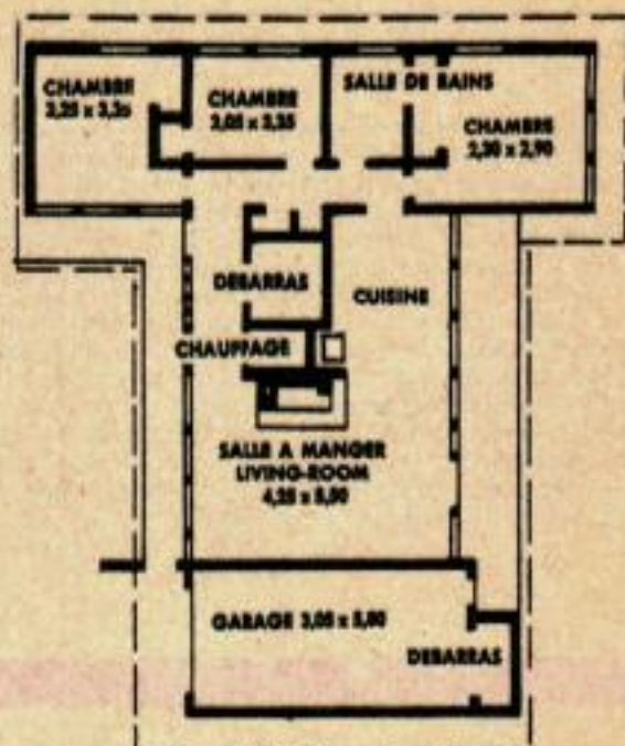
Les grandes baies de la façade postérieure de cette maison donnent sur un patio ouvert. Le garage est à gauche. L'aile des chambres à coucher à droite.
