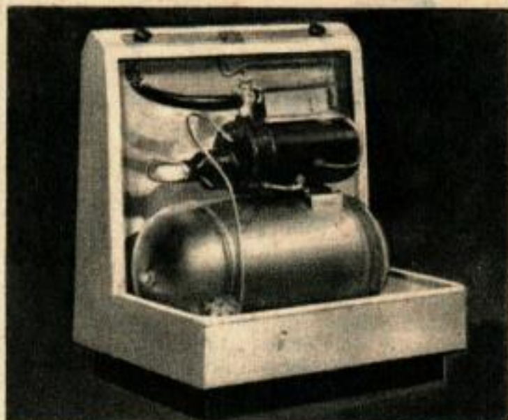
1. Cette installation d'eau sous pression est contenue dans un meuble de cuisine rutilant. Une pompe entraînée par un moteur électrique montée sur le réservoir de 45 litres débite jusqu'à 3 000 litres à l'heure. Ce groupe est la seule installation de pompage nécessaire pour tirer l'eau d'un puits dont la profondeur peut être comprise entre 7,50 m et 25 m. L'indicateur et le commutateur sont montés sur un tableau de commande.
